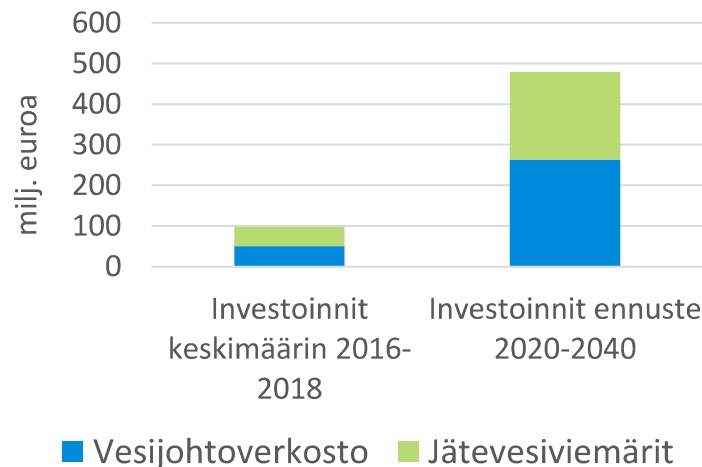
Verkostosaneeraus vuotuinen investointi ja investointitarve
