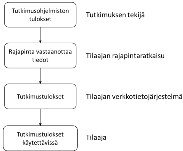
Kuva 4.3. Verkostotutkimuksen tulokset
