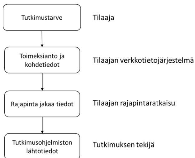
Kuva 4.2. Verkostotutkimuksen tilaaminen
